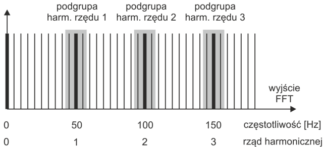
Rys. 15. Wyznaczanie podgrup harmonicznych (sieć 50 Hz).
